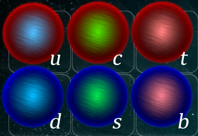
Quarks
