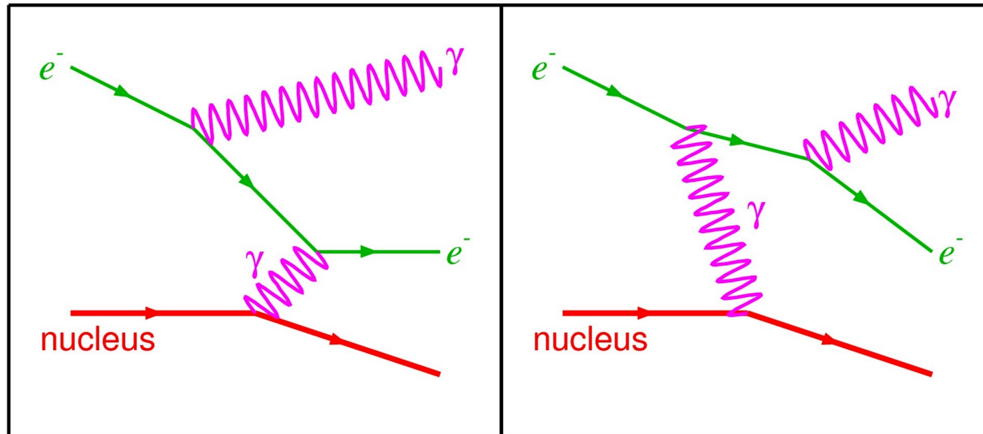
Bremsstrahlung
