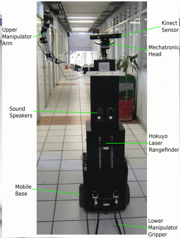
Robot AL-ITA (2011)
