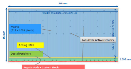
ALPIDE chip
