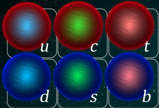
Quarks
