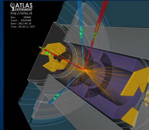
ATLAS
