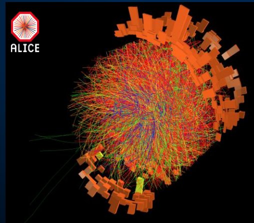
ALICE
