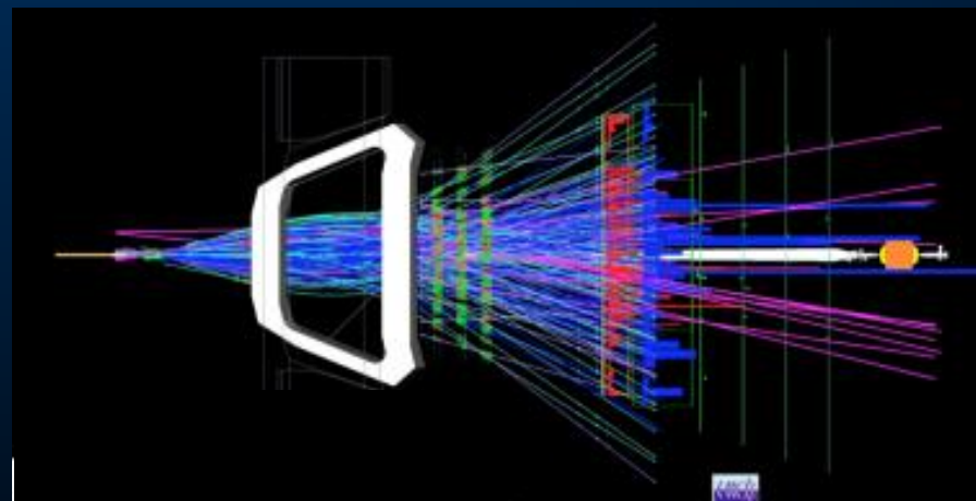
LHCb
