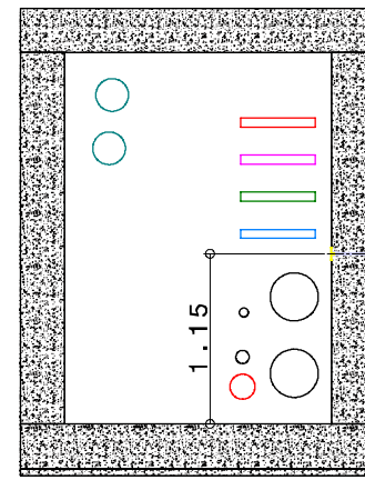
D-D 1:20
