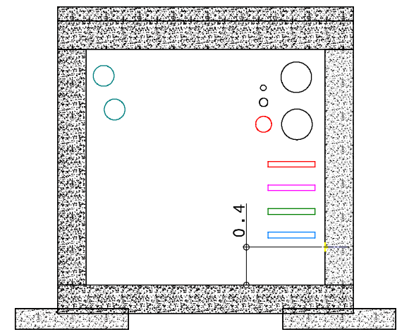
E-E 1:20
