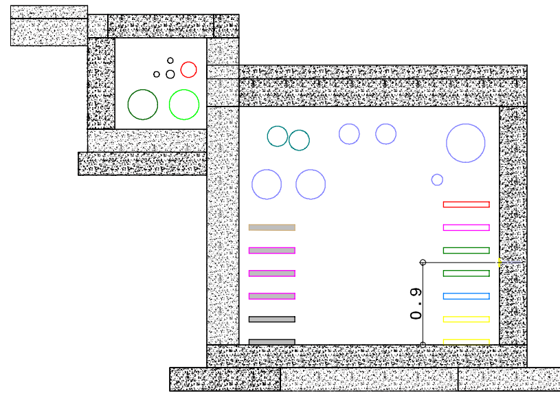
F-F 1:20
