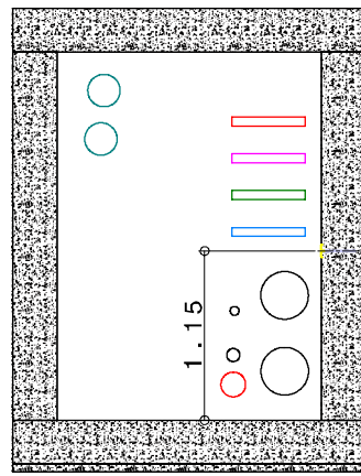
C-C 1:20
