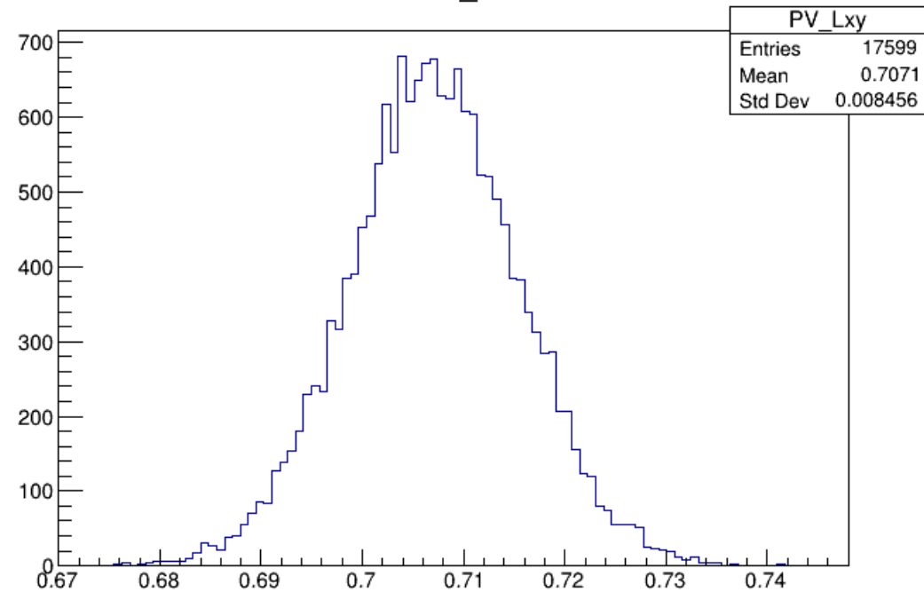
PV_r
