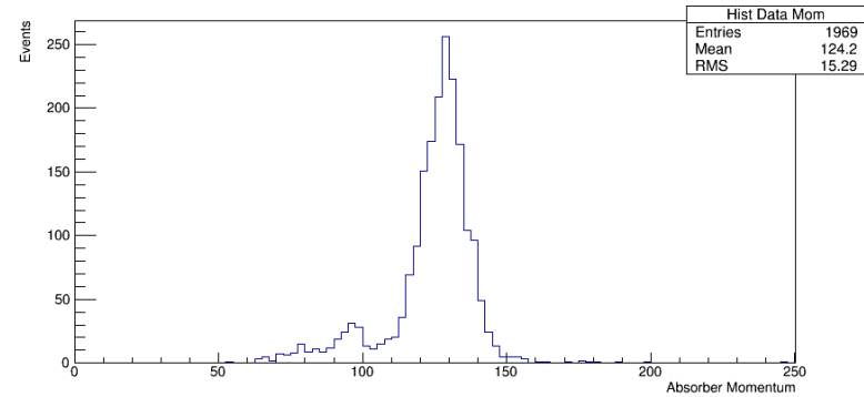
Momentum
