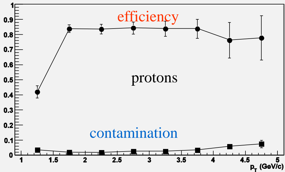
Protons
