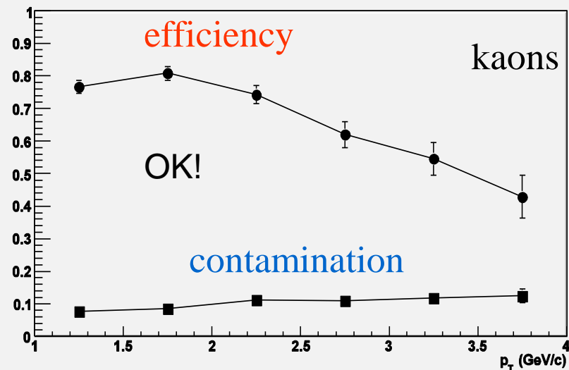
Kaons
